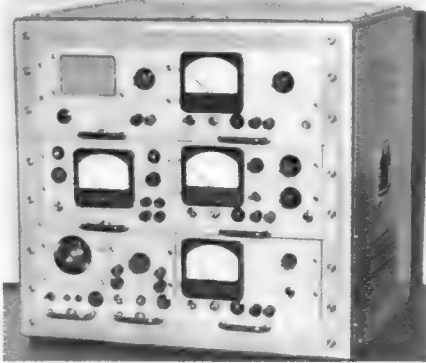
Service-Meßplatz nach dem Einschubsystem von der Firma G. Haeberlein. Die Einschübe sind dem genormten 19-Zoll-System angepaßt. Man kann den Meßplatz somit für spezielle Aufgaben leicht umrüsten
