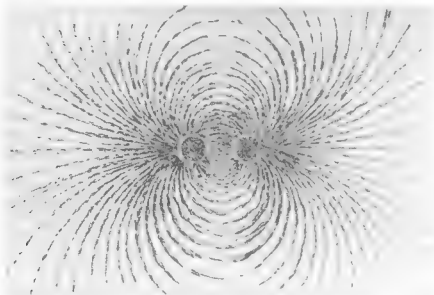
Bild 3. Magnetisches Induktionsfeld der 1-kHz-Spule
