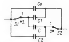
Rechts: Bild 10. Kondensatoren des Hochpasses
