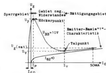
Statische Emittiercharakteristik mit den wichtigsten Parametern und Messpunkten (stark idealisierte Darstellung)
