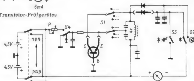
Bild 2. Schaltung des dynamischen Transistor-testers Semitest II
