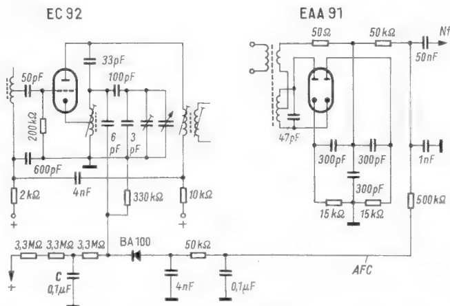
Ein Feinschluß des Siebkondensators C veränderte die Vorspannung der Nachstimm-diode und führte zu einem sprunghaften Wechseln der Oszillatorfrequenz
