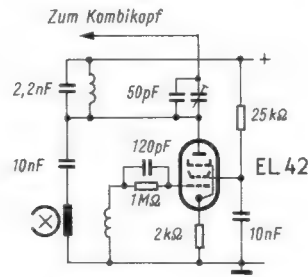
Bild 2. Abgeänderter Hf-Oszillator
