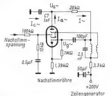
Bild 20. Nachstimmenschaltung des Zeilengenerators
