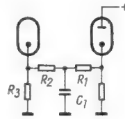
Rechts: Bild 5: Prinzip der Aufsprech-Entzerrung
