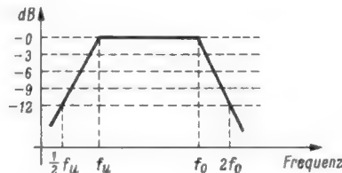
Bild 3. Ideale Kennlinie eines kombinierten Hoch- und Tiefpaßfilters
