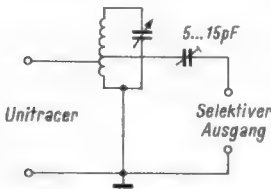
Bild 4. Durch Anschalten eines Abstimmkreises kann ein enges Band aus dem Frequenzgemisch herausgesiebt werden
