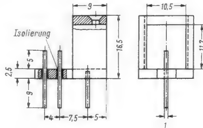
Bild 6: Konstruktion des Kopfhalters
