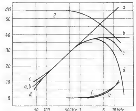
Bild 3. Kurven für den Tonkopf MK 100, v = 9,5 cm/sec. a = \omega -Gerade, b = Kurve des idealen Hörkopfes (konstruiert aus a minus g), c = Wiedergabe mit DIN-Normband, d = Wiedergabe der Aufnahme mit konstantem Aufsprichstrom, e = erforderliche Höhenanhebung bei Aufnahme (konstruiert aus c minus d), f = durch RC-Glied erzielte praktische Kurve e, g = Bandflußkurve für \tau = 100 µsec nach Gleichung (1)
